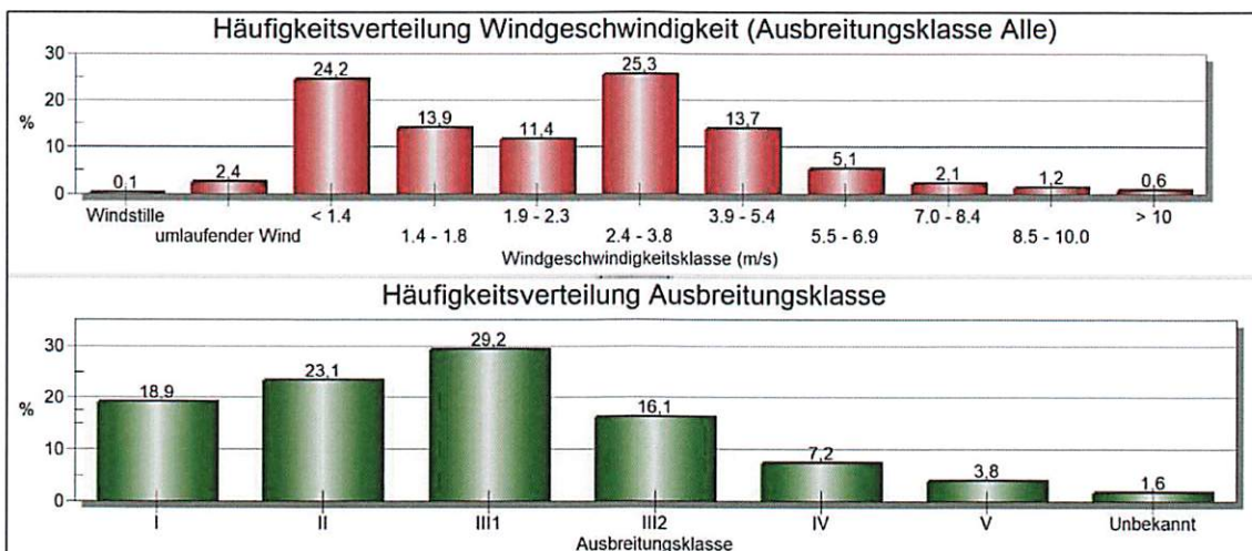
Abbildung 19: Häufigkeitsverteilung der Windgeschwindigkeiten und Ausbreitungsklassen (München-Flughafen 2014) /15/
