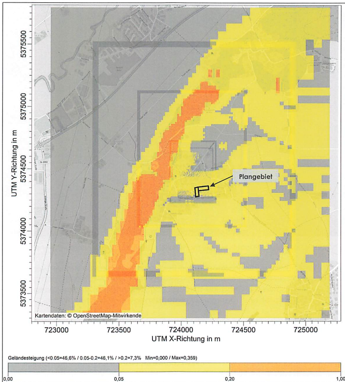
Abbildung 14: Lageplan mit Darstellung der Geländesteigungen im Plangebiet
