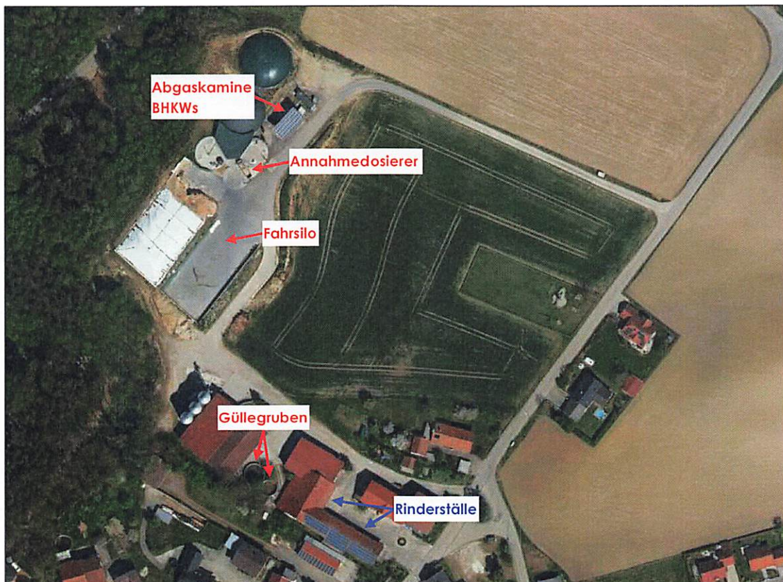
Abbildung 10: Luftbild mit Darstellung der Emissionsquellen der Rinderhaltung und der Biogasanlage /19/
